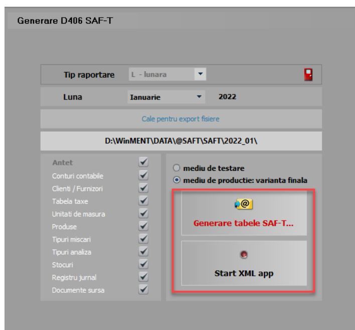
Macheta pentru Generare tabele SAF-T si deschidere XML
